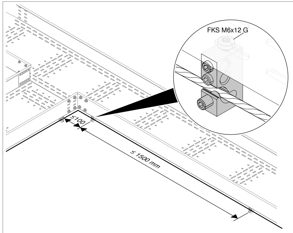
Abb. 12: Befestigung Anschlussklemme aufgeständertes System
