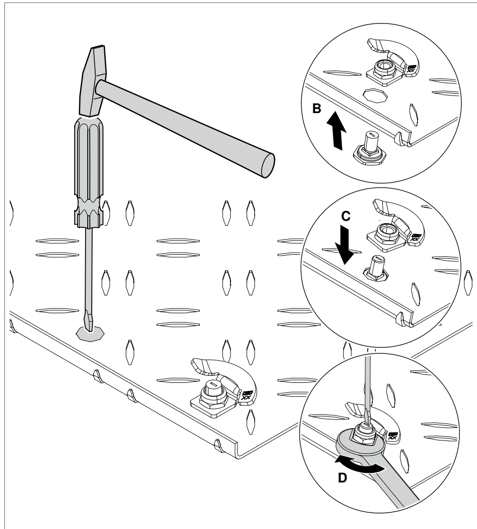
Abb. 20: Montage Drehriegel Typ DRL H S FT
