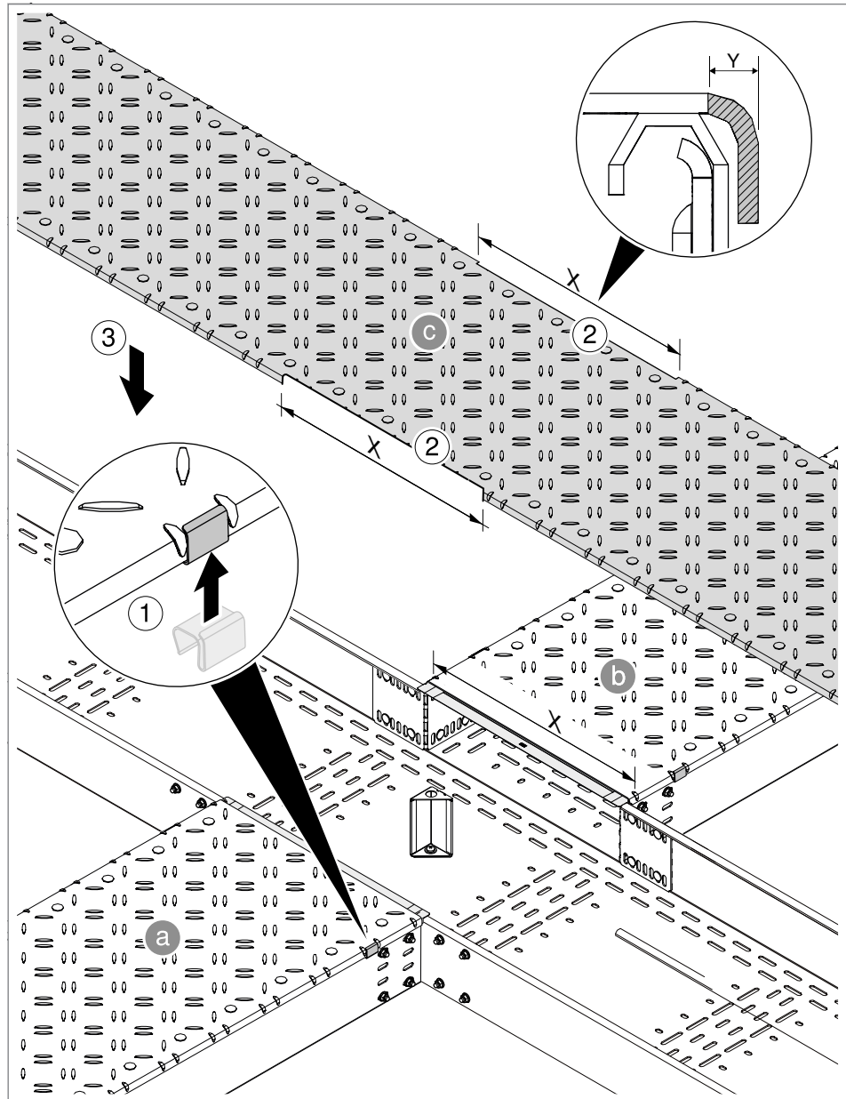
Abb. 23: Montage Deckel bei Kreuzverbindung
