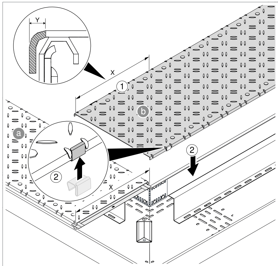
Abb. 22: Montage Deckel bei Eckverbindung
