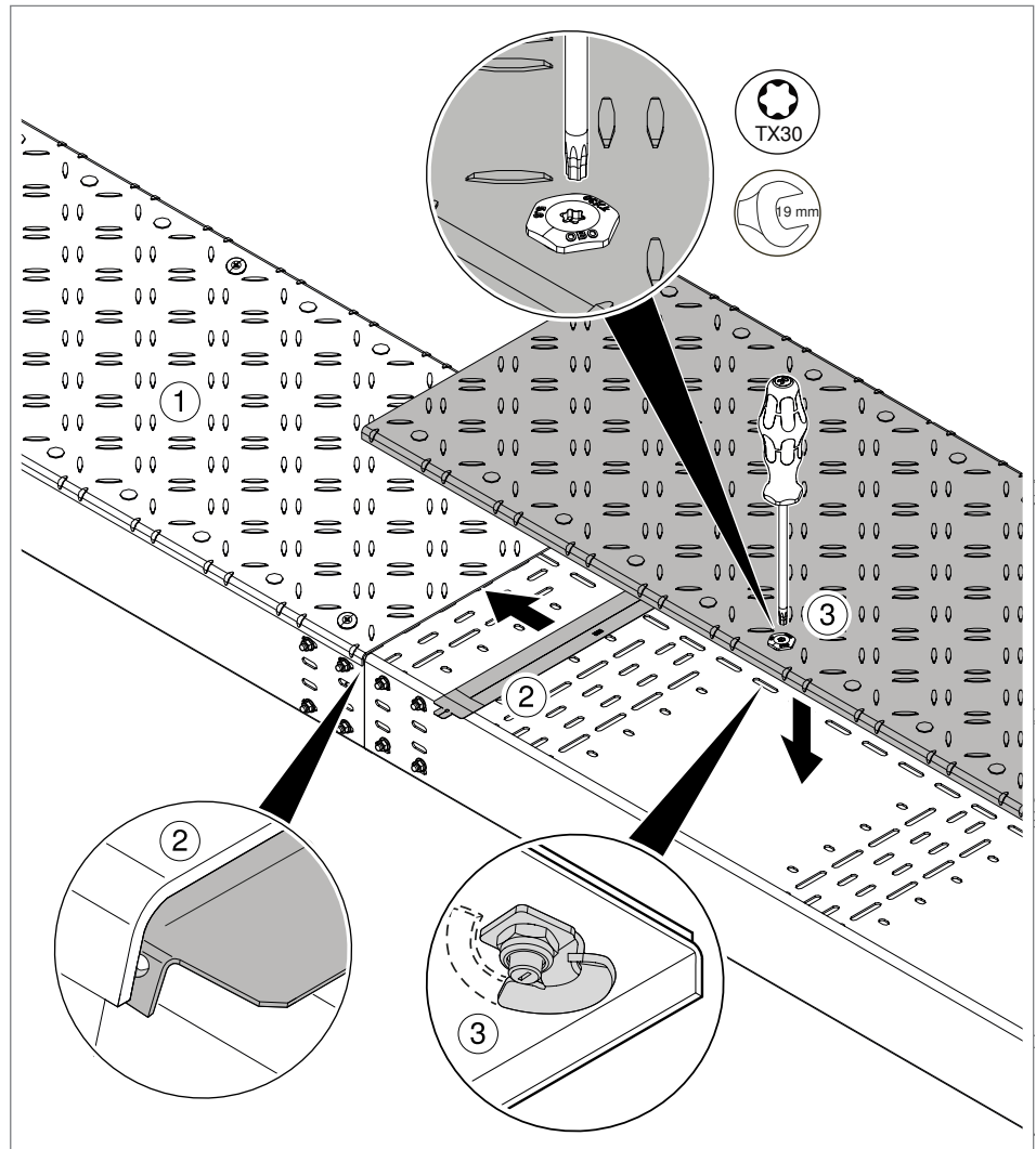
Abb. 21: Montage Deckeltyp DBKR mit Drehriegel
