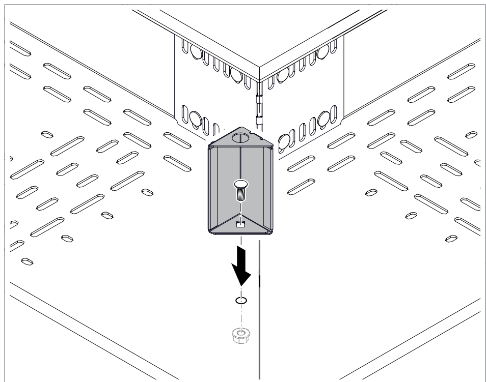
Abb. 17: Montage Deckelstütze
