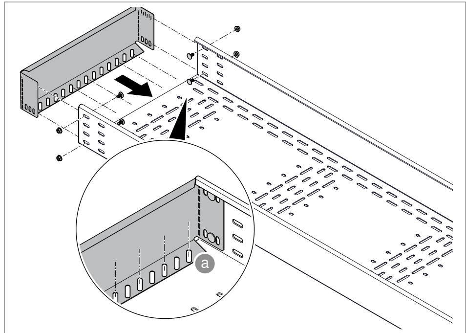
Abb. 10: Abschluss offene Enden
