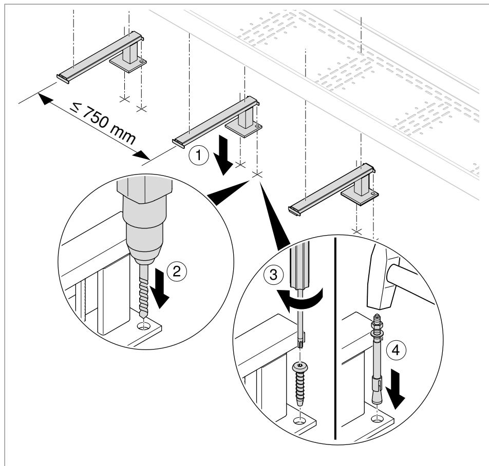
Abb. 4: Montage Stützausleger
