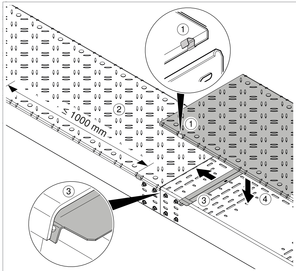
Abb. 19: Montage Deckel DBKR mit Deckelklammern
