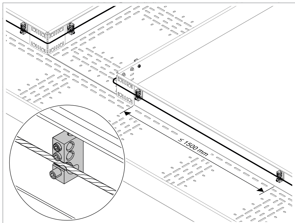
Abb. 14: Abstand Anschlussklemme, System auf Profilschiene („Montage“)
