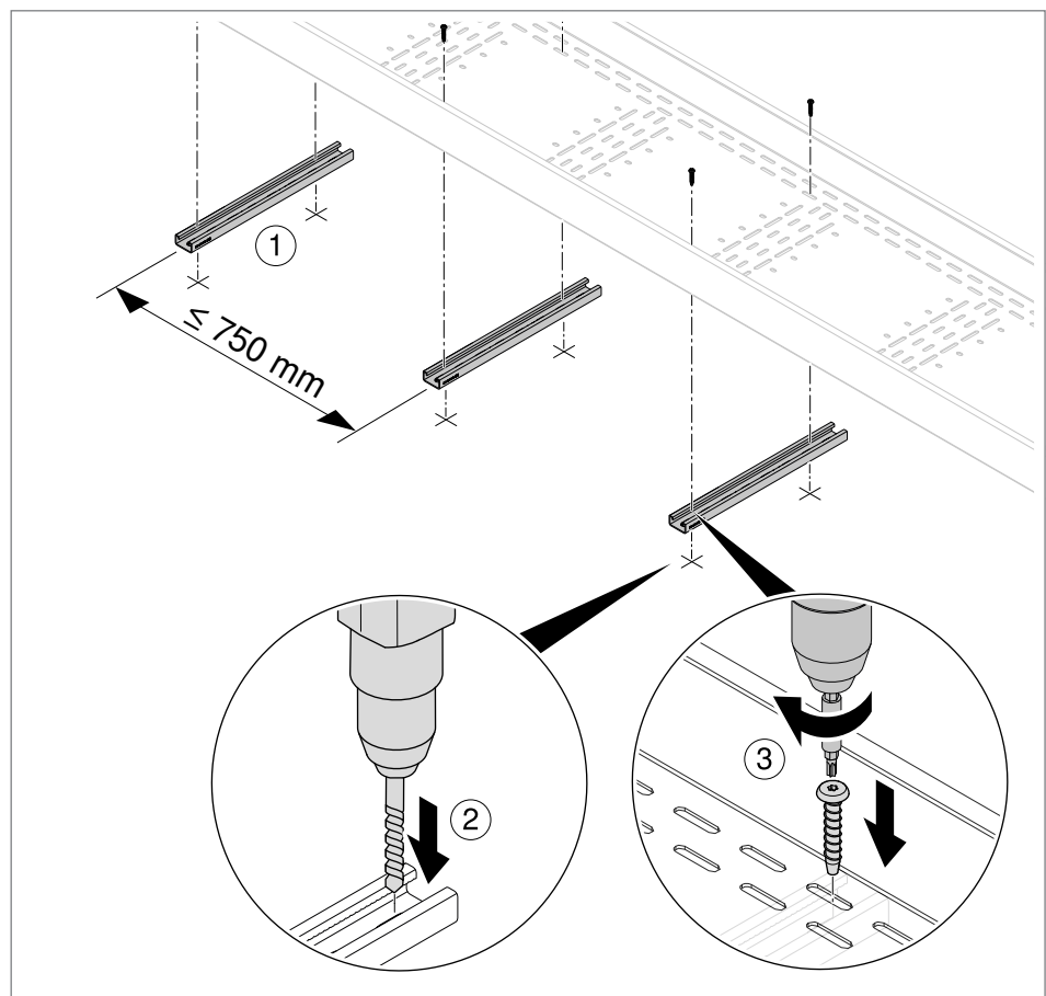
Abb. 3: Montage Profilschiene
