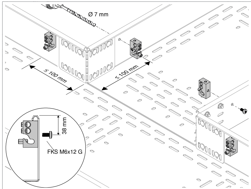
Abb. 13: Befestigung Anschlussklemme System auf Profilschiene („Montage“)
