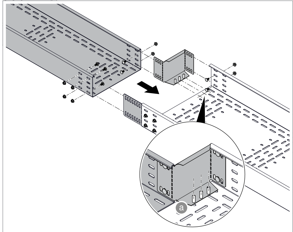
Abb. 9: Veränderung Rinnenbreite
