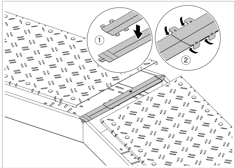
Abb. 18: Montage Staubschutzelement mit Verlängerung
