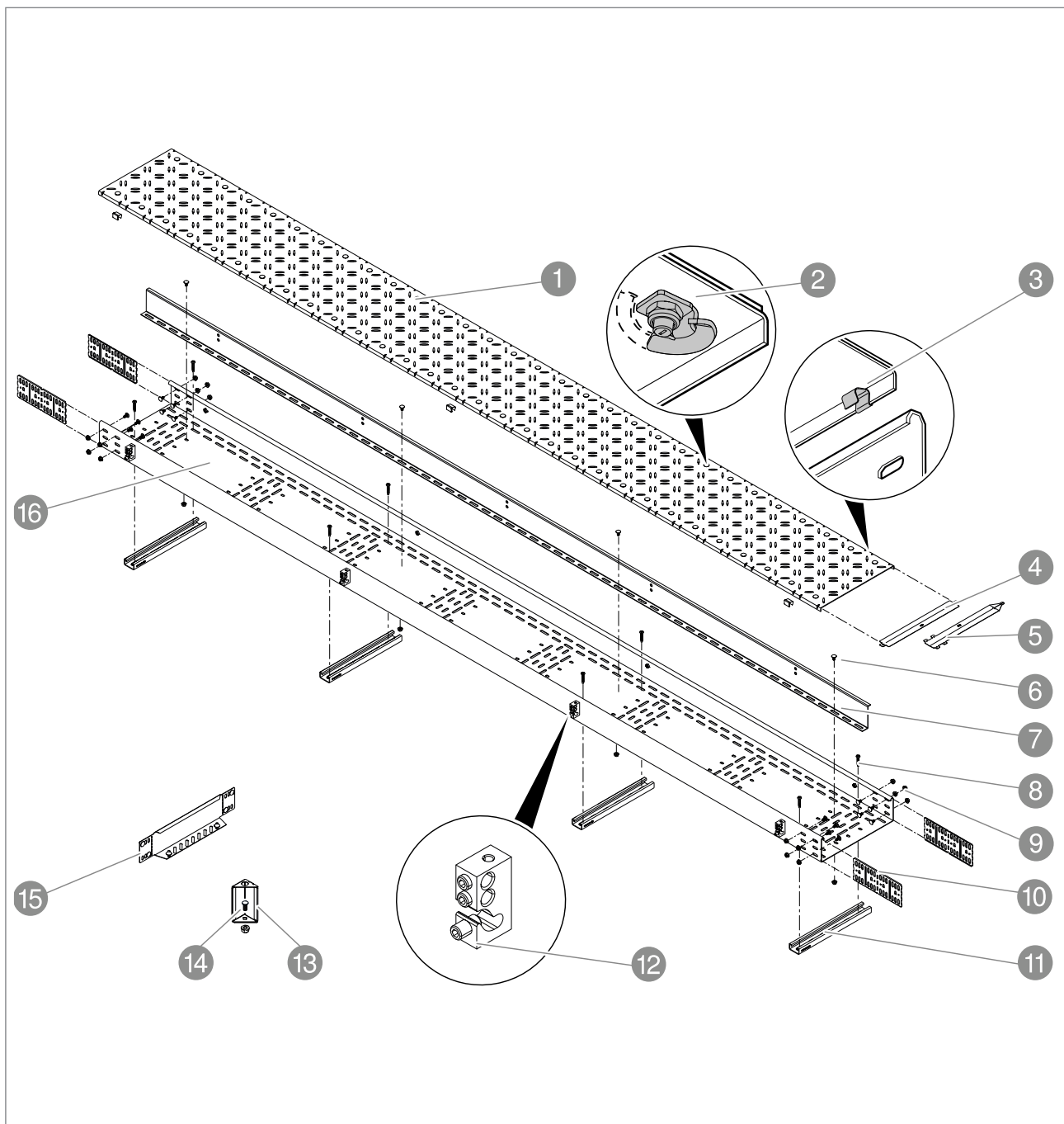
Abb. 2: Systemkomponenten Fördertechnikrinne, nicht begehbar
