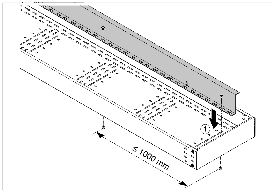
Abb. 11: Trennstegmontage
