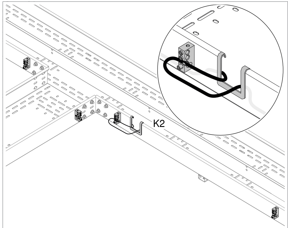
Abb. 16: Abstand Anschlussklemme, System auf Profilschiene („Fördertechnik“)
