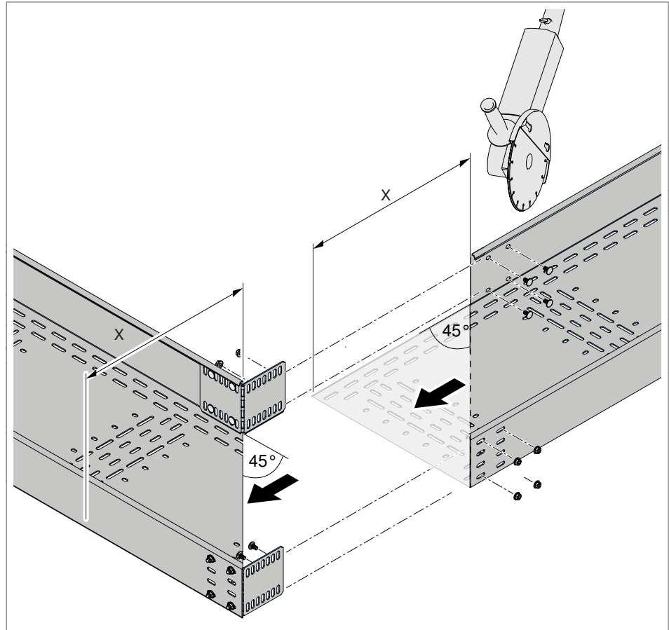
Abb. 7: Eckverbindung
