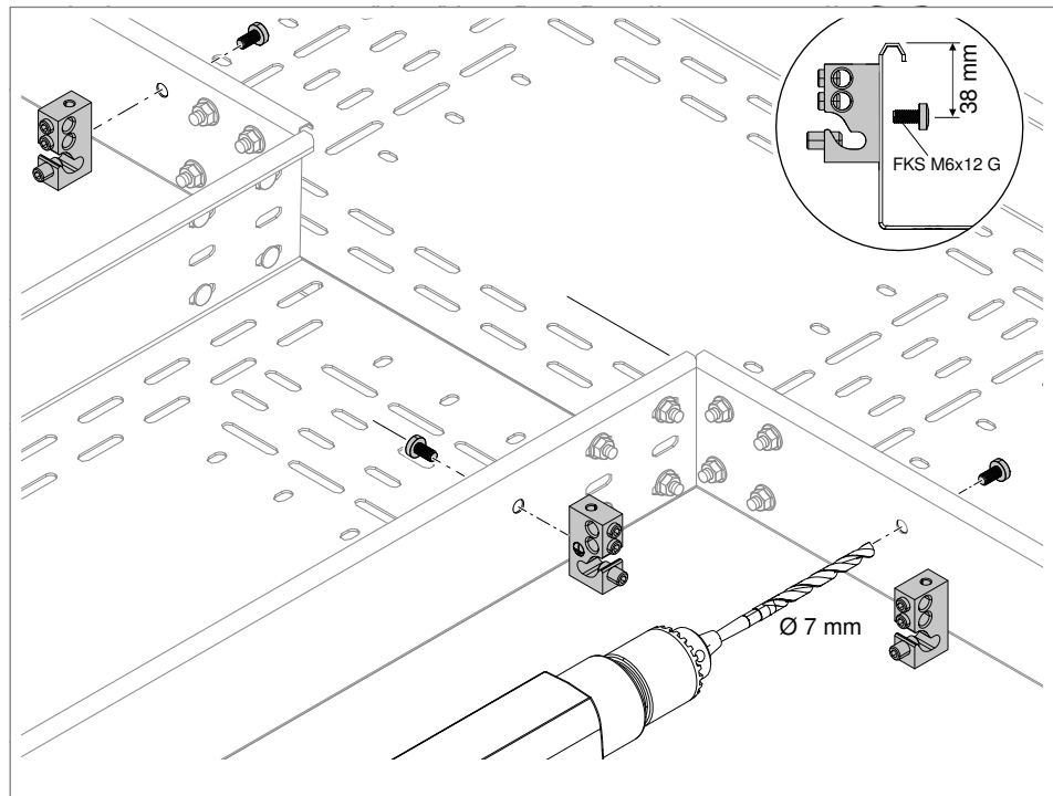
Abb. 15: Befestigung Anschlussklemme, System auf Profilschiene („Fördertechnik“)
