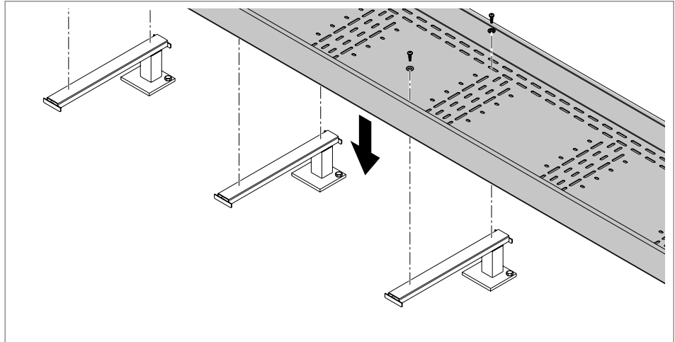
Abb. 5: Montage auf Stützauslegern
